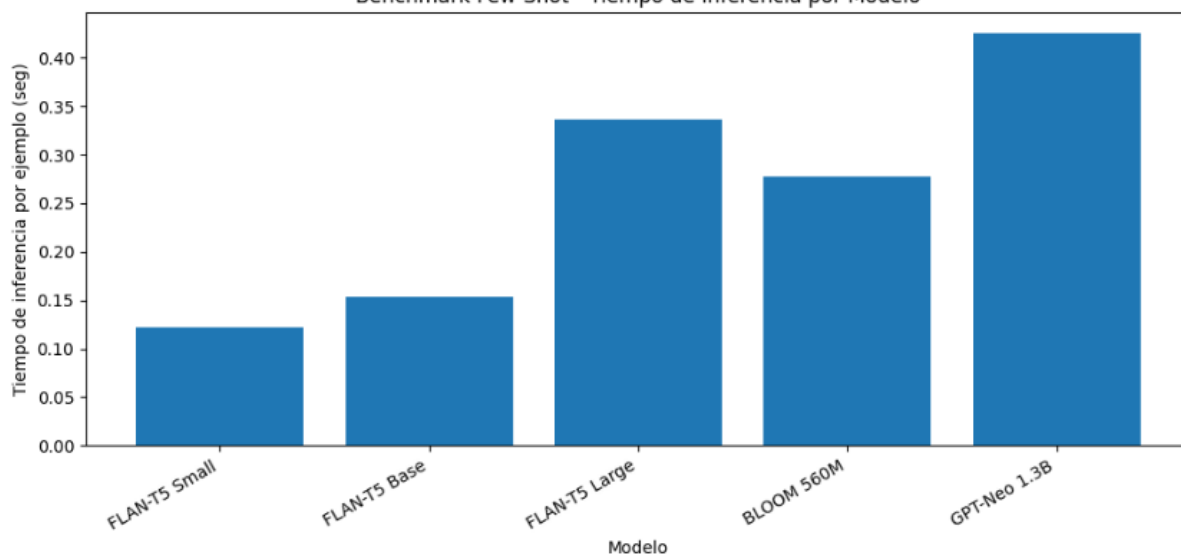
*** Benchmark Few-Shot - Tiempo de Inferencia por Modelo
